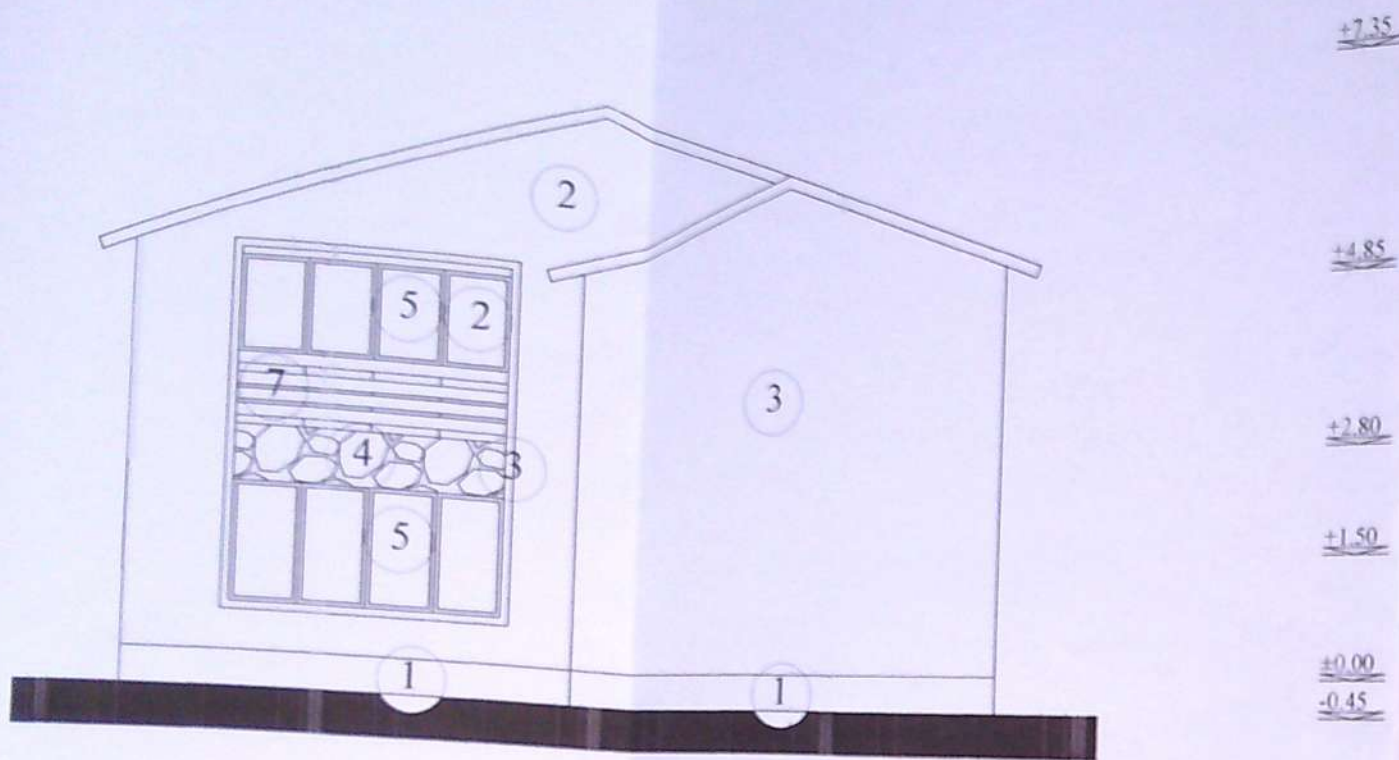
FATADA SUD
